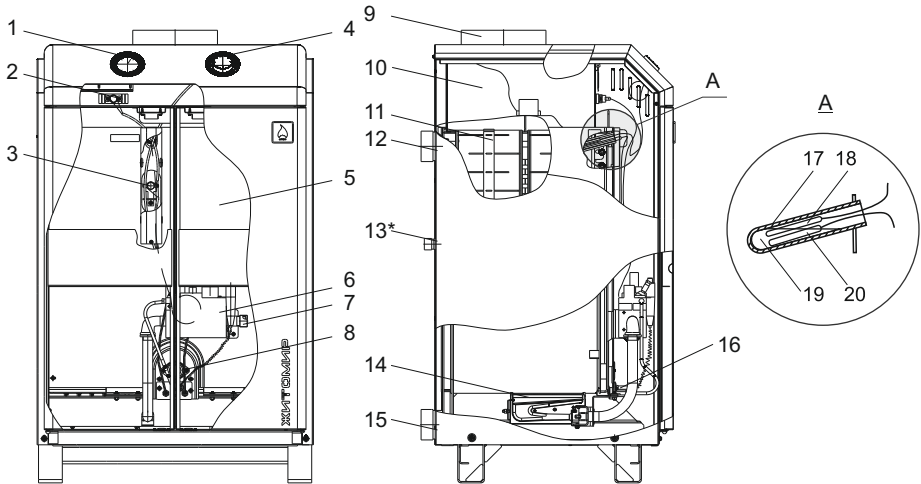
Рис. 1а. Схема конструкции котла 80 кВт (декоративный кожух не показан)
